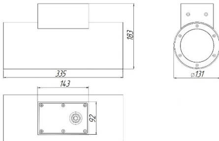
Рисунок 1 Светильник «L-facade x2»
